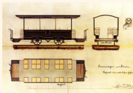
nákres jednoho z vozů koněspřežné dráhy
